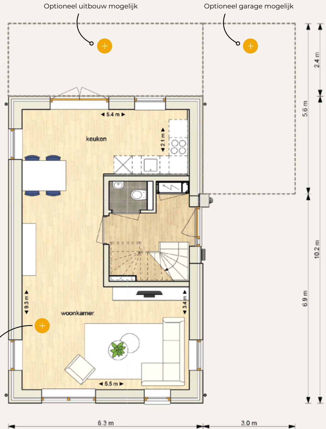
Begane grond
