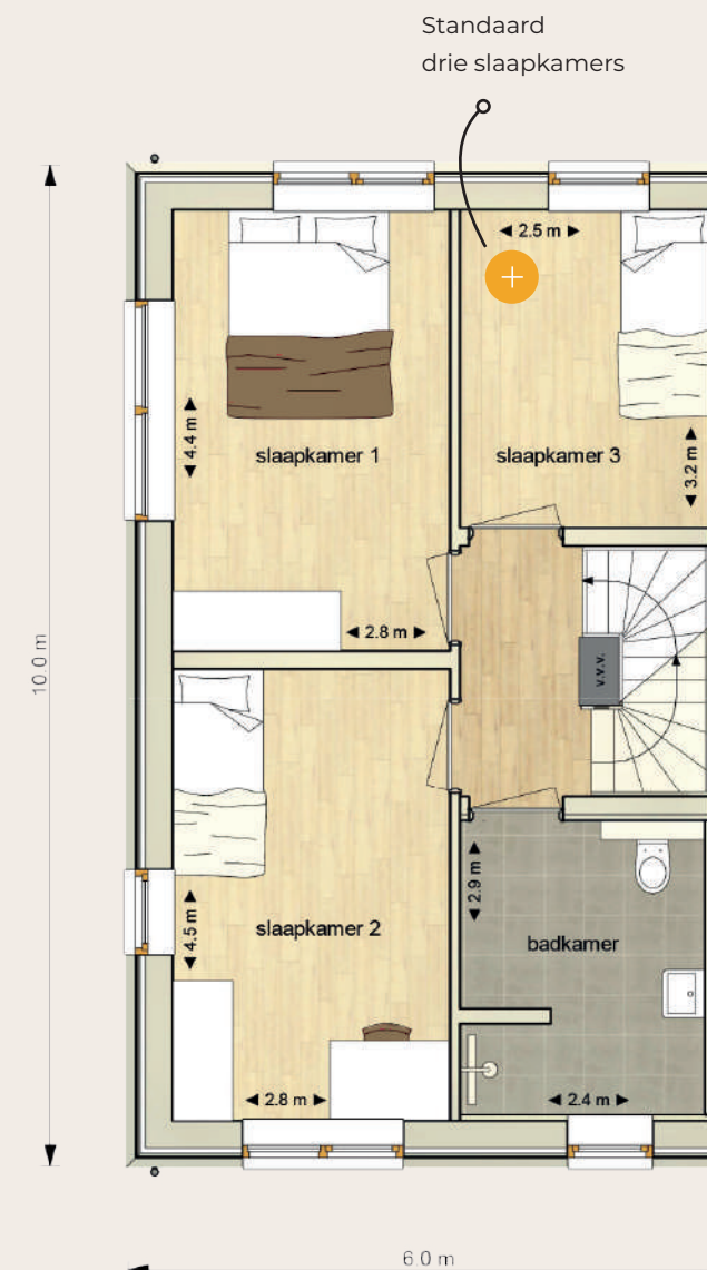
Verdieping
