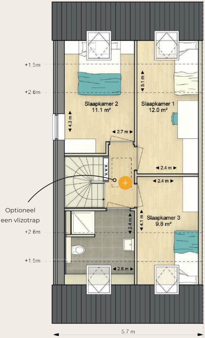
Verdieping
